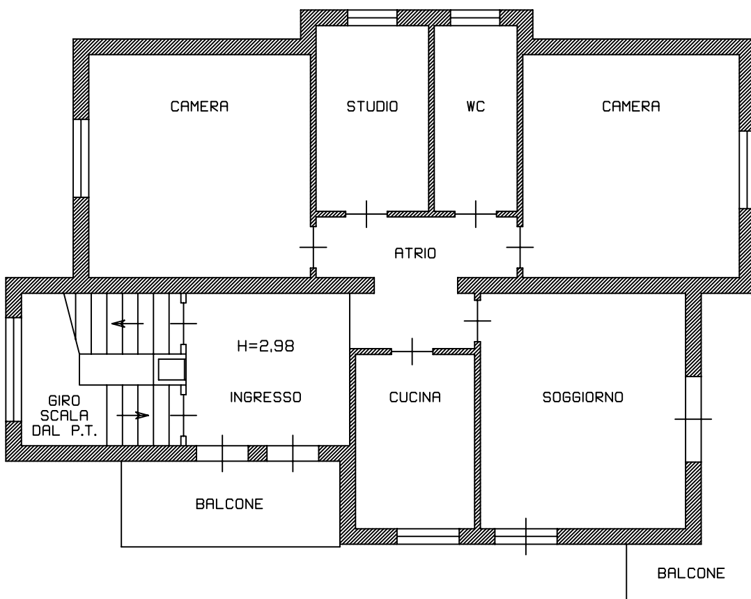
SITUAZIONE ESISTENTE PIANO PRIMO
