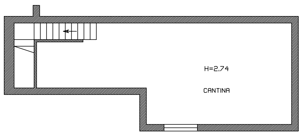
SITUAZIONE CATASTALE PIANO INTERRATO
